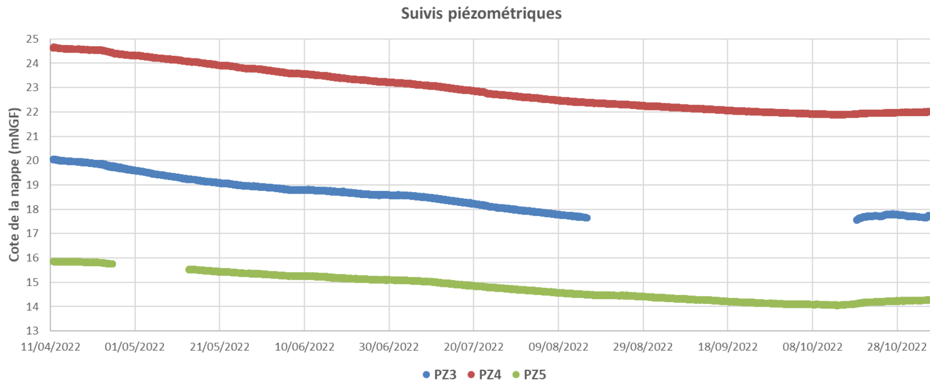
Figure 7. Suivis piézométriques au droit de PZ3, PZ4 et PZ5 du 11/04/2022 au 04/11/2022
