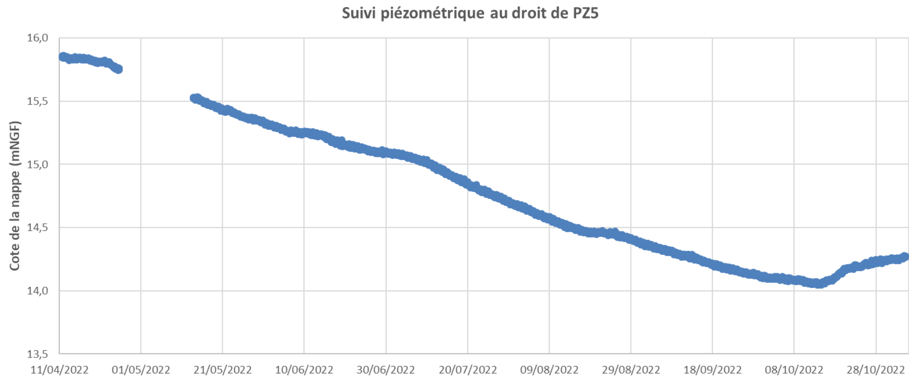
Figure 6. Suivi piézométrique au droit de PZ5 du 11/04/2022 au 04/11/2022
