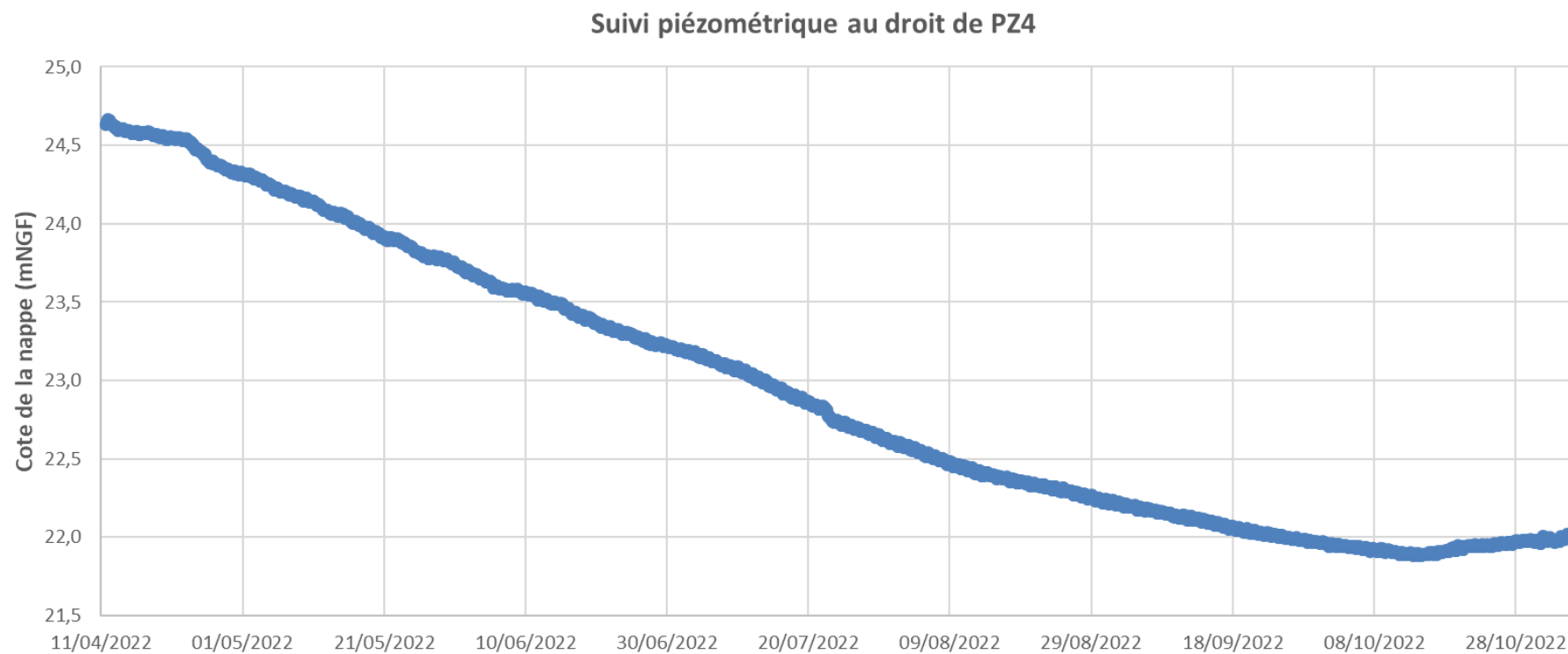
Figure 5. Suivi piézométrique au droit de PZ4 du 11/04/2022 au 04/11/2022
