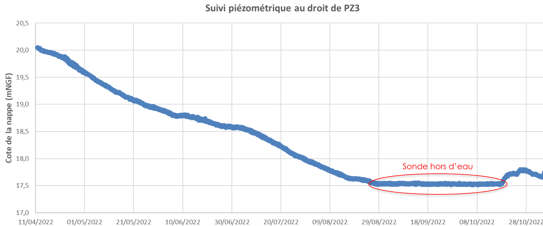
Figure 4. Suivi piézométrique au droit de PZ3 du 11/04/2022 au 04/11/2022
